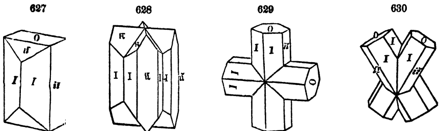
cruciform: twinning-plane i\bar{i} (f. 628); \frac{1}{2}I (f. 629); and \frac{1}{2}I (f. 630). Fig.
